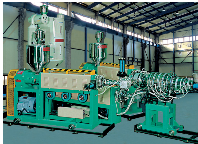
EXTRUDERS & DIE
